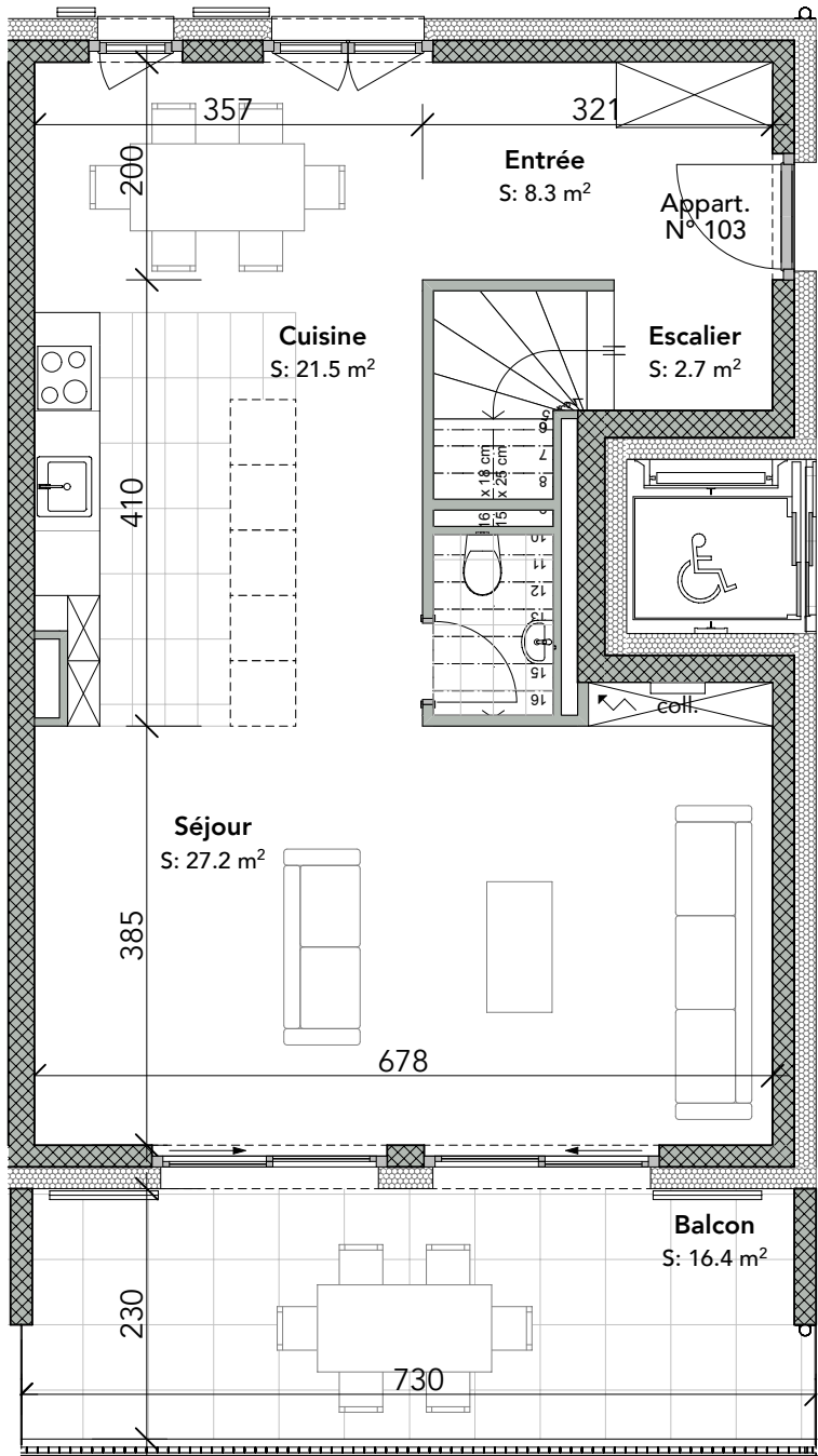
PLAN 1er ETAGE
